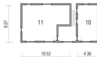
Planta Piso 1 . esc: 1/500
